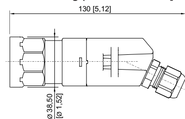
8003/...-726 Drehgriff
