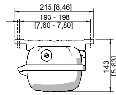
Montageschiene
