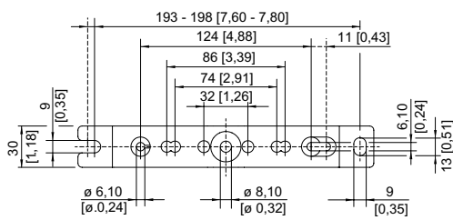
Montageschiene
