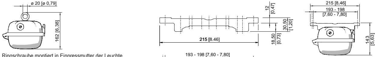
Montageschiene
