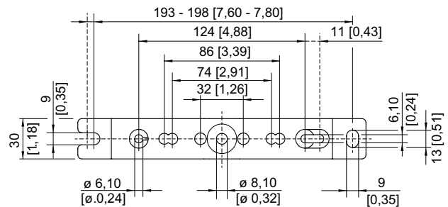
Montageschiene
