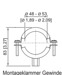
Montageklammer Gewinde
