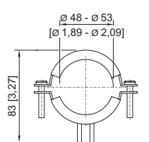
Montageklammer Gewinde
