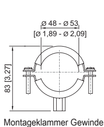
Montageklammer Gewinde
