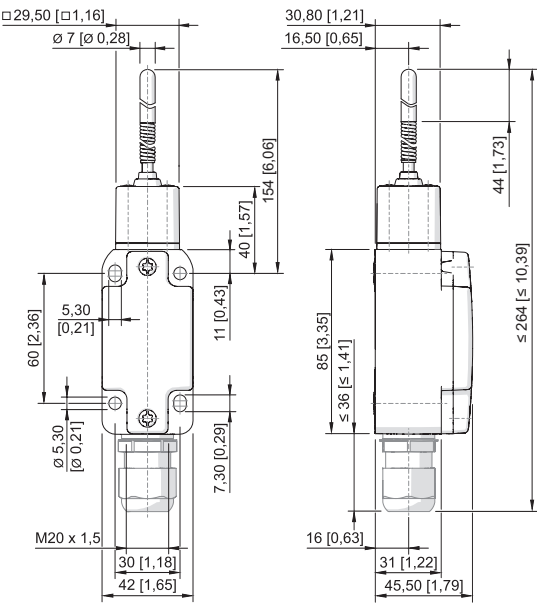
Federstab 8070/2-.-TK-U60
