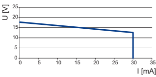
输出特性曲线 9475/32-08-52, 9475/33-08-50
