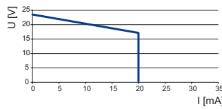
输出特性曲线 9475/32-08-62, 9475/33-08-60
