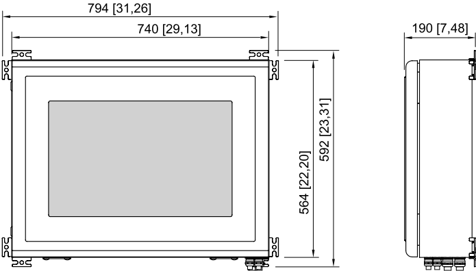
工作站 FR 箱体，壁挂式安装
