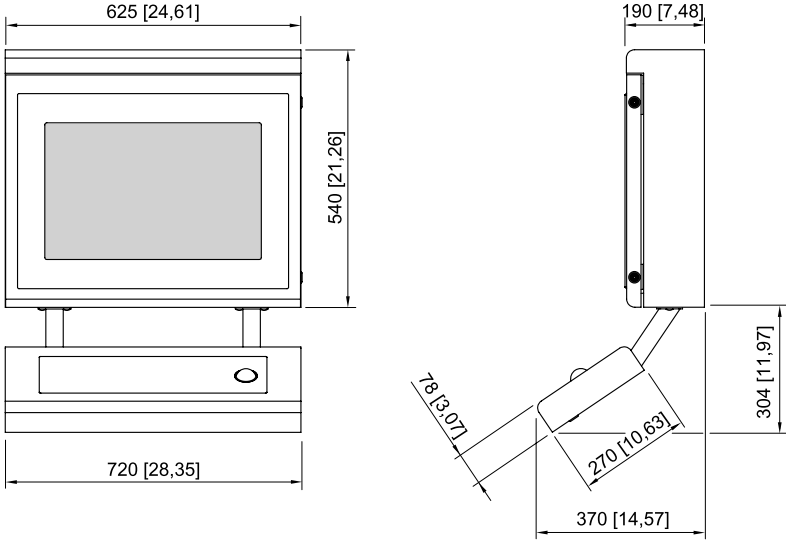
工作站 CFR 箱体
