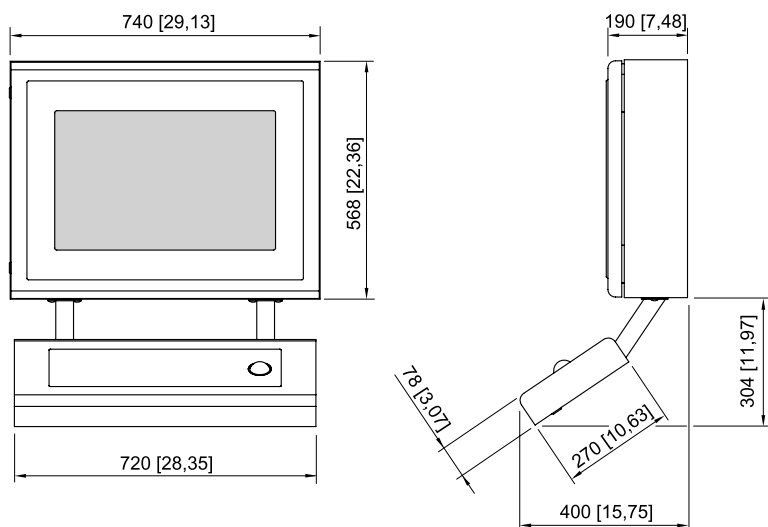
操作站 FR 箱体
