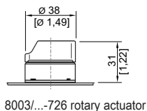
8003/...-726 rotary actuator
