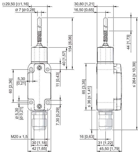
Spring rod 8070/2-2-TK-U60
