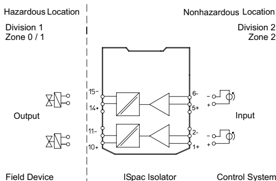
Connection diagram 9176/20-...
