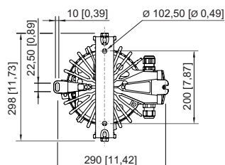
Avec étrier de montage
