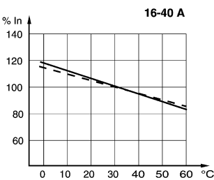
Facteurs de correction pour les températures ambiantes différentes de 30 °C
