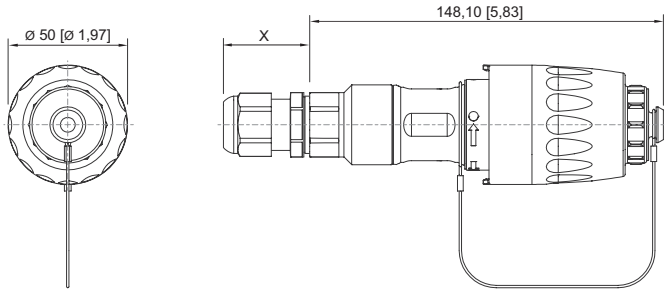
8595/1 Fiche X = en fonction du presse-étoupe utilisé
