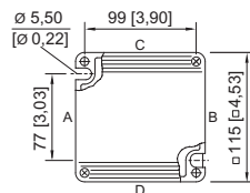
8118/.2. Boîtier taille 2
