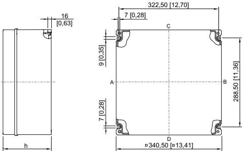
Plan d'encombrement (toutes les dimensions sont en mm [pouces]) – sous réserve de modifications
