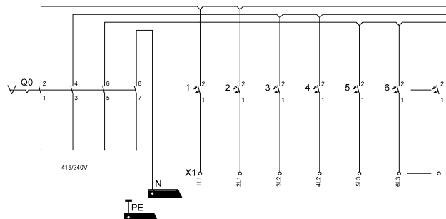
Schéma de connexion 8146/5-ExV-...-.....1P-T
