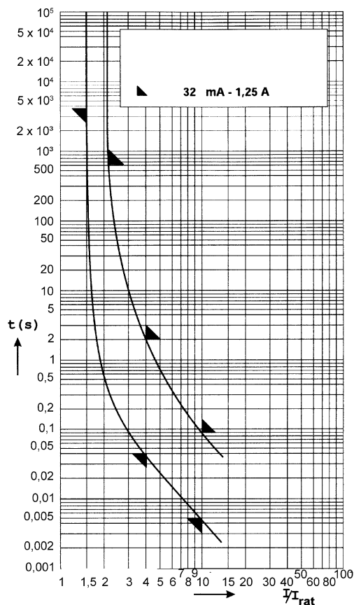
8560/51-...1, 250 V, semi-temporisé
