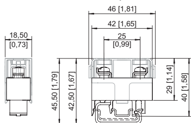
8560/51-...1, 250 V, semi-temporisé
