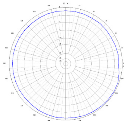
Caractéristiques de rayonnement pour 2,4 GHz Type 9790/1-2458-NT.-53
