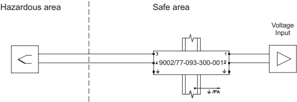
Cas d'application : thermocouples
