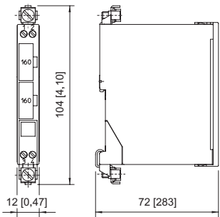
Barrières Zener de sécurité intrinsèque deux canaux, potentiel : + / +
