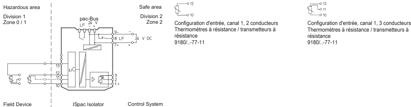
Schéma de raccordement 9180/1.-77-11
