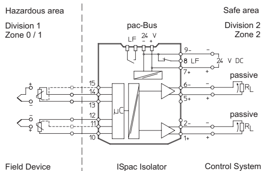
Schéma de raccordement 9182/20-51-11
