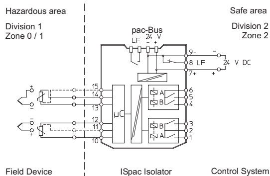
Schéma de raccordement 9182/20-50-12
