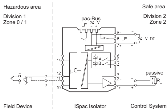
Schéma de raccordement 9182/10-51-12 ; 9182/10-51-14
