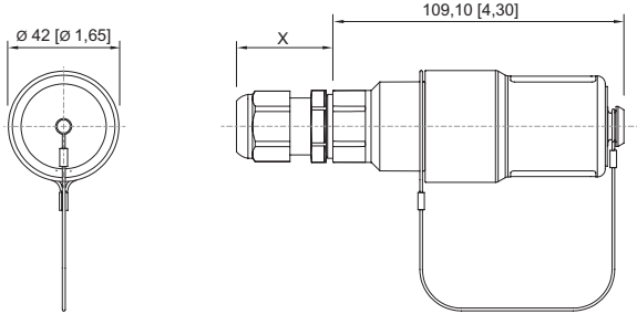
8595/1 Accouplement X = en fonction du presse-étoupe utilisé
