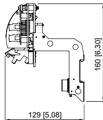
Support de bus 9419/04R pour 4 segments de bus de terrain
