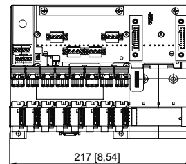
Support de bus 9419/04R pour 4 segments de bus de terrain
