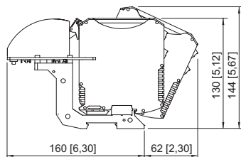
Support de bus 9419 avec modules
