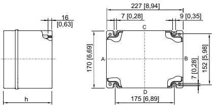
Plan d'encombrement (toutes les dimensions sont en mm [pouces]) – sous réserve de modifications
