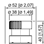
8003/...-010, 8003/...-012 Bouton d'arrêt Ø 38 mm
