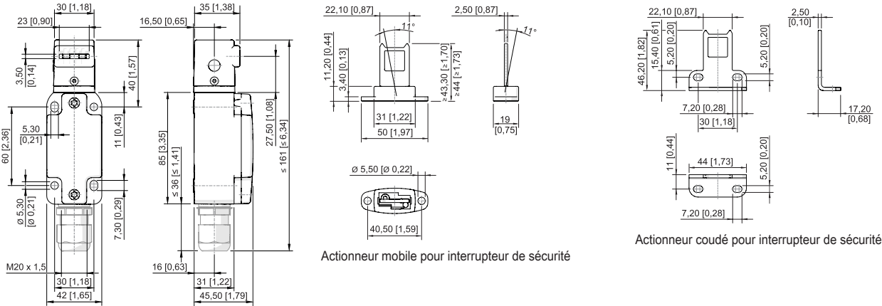
Interrupteur de sécurité 8070/2--AZ-U50
