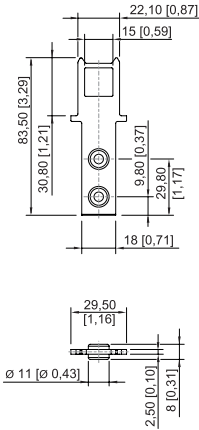
Actionneur droit pour interrupteur de sécurité
