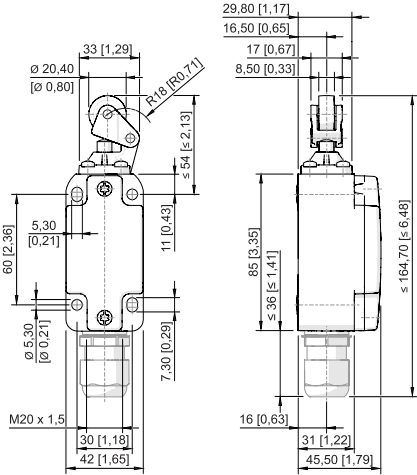
Levier à galet 8070/2-3-WH-U60
