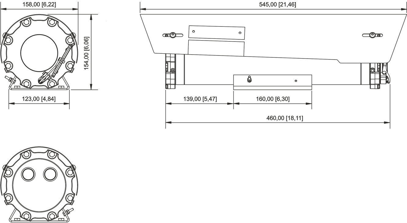
Plan d'encombrement (toutes les dimensions sont en mm [pouces]) – sous réserve de modifications
