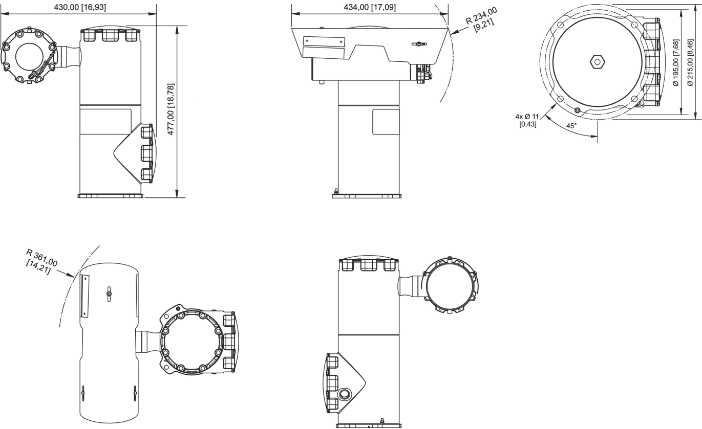
Plan d'encombrement (toutes les dimensions sont en mm [pouces]) – sous réserve de modifications
