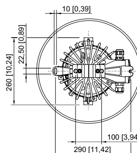
Avec dispositif anti-éblouissement et collier de serrage
