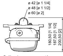
Collier de serrage monté sur support rail DIN
