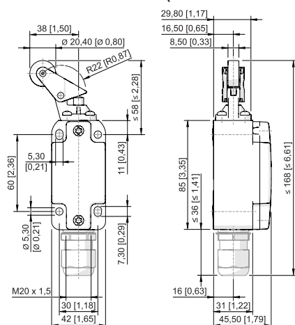
Levier à galet 8070/2-3-WPH-U60
