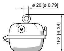
Vis à œil montée dans l'écrou à servir du luminaire
