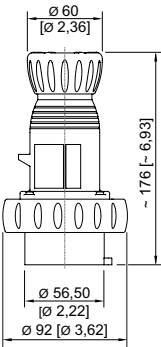
Fiche 5 pôles
