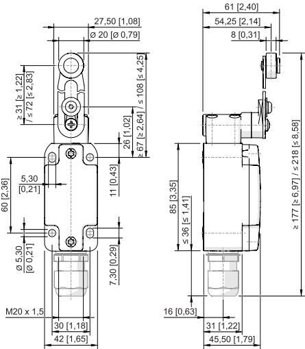
Levier pivotant 8070/2--DS-U60
