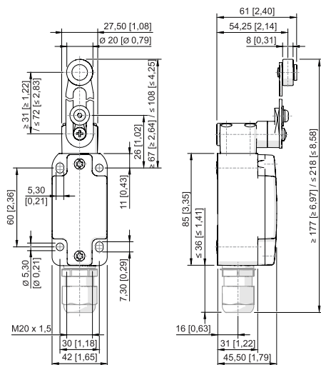
Levier pivotant 8070/2-5-DS-U60
