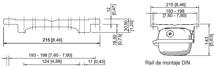
Raíl de montaje DIN
