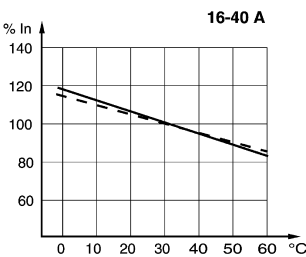
Factores de corrección para temperaturas ambiente distintas de 30 °C
