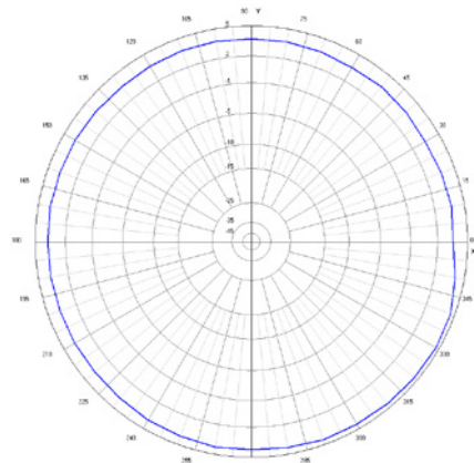
Características de radiación para 2,4 GHz Tipo 9790/1-2458-NT.-53
