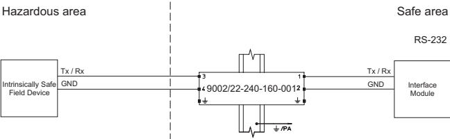
Caso de aplicación con RS 232
