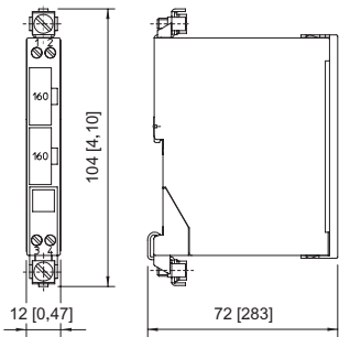
Barreras de seguridad intrínseca de dos canales para potencial ~/~
