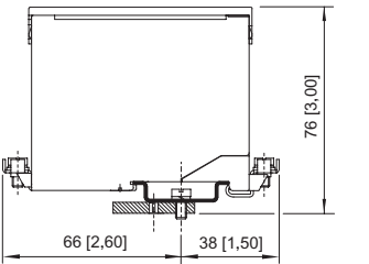
Montado en placa de montaje con adaptador
