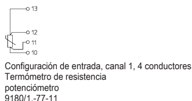
Diagrama de conexión 9180/1.-77-11
