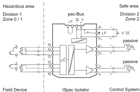
Esquema de conexiones 9182/20-51-11
